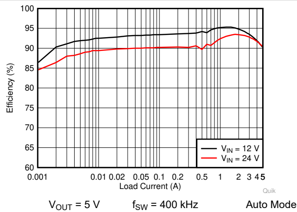
图 8-4. LM76005 Efficiency
