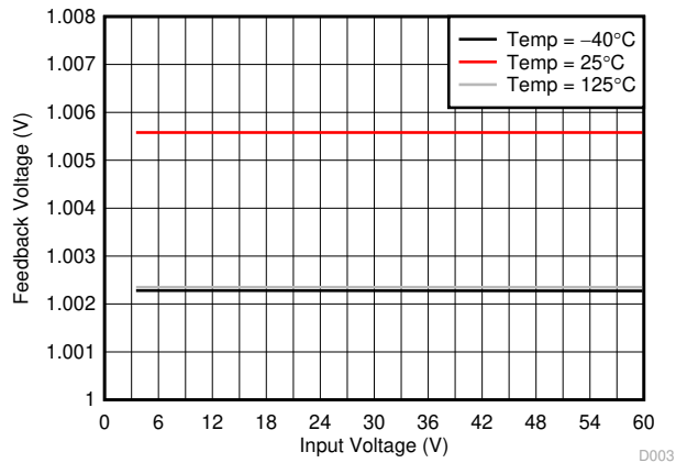
图 6-3. Feedback Voltage
