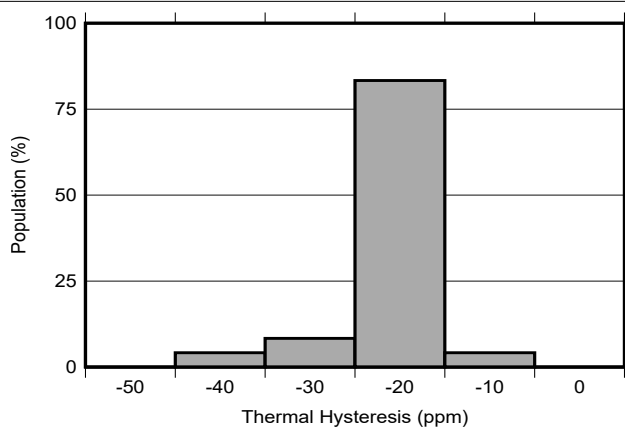
图 6-49. 热磁滞分布：周期 2 ( -40^\circ\text{C} 至 125^\circ\text{C} )
